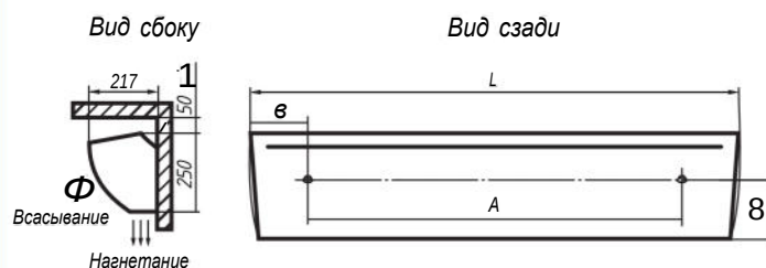
Вид и габариты ТЗВ-804, 5/22, ТЗВ-1000/25, ТЗВ-1400/25 «Иртыш»
