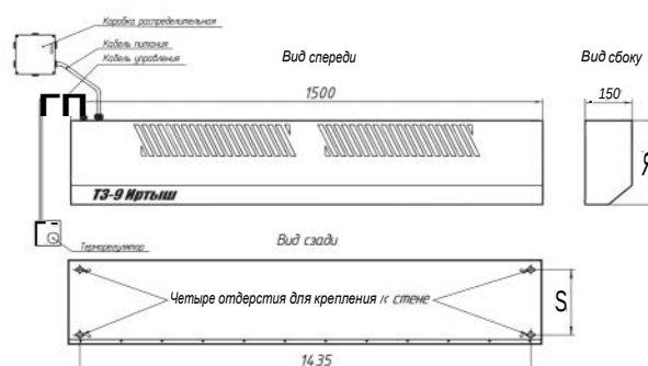
Вид и габариты Т3-9, Т3-12 «Иртыш»
