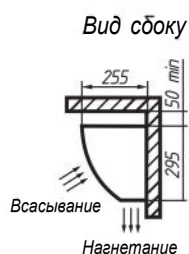
Вид и габариты ТЗВ-1000/40, ТЗВ-1400/40, ТЗВ-1900/30-40 «Иртыш»
