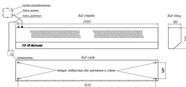
Вид и габариты ТЗ-15, ТЗ-18 «Иртыш»
