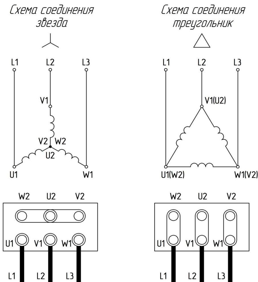
Рис. 2 Схемы подключения питания для трехфазного асинхронного двигателя
