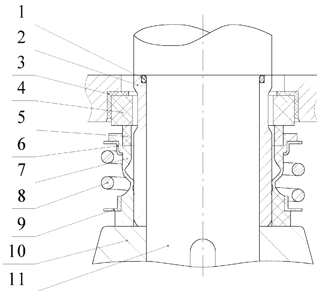
Рис. 4. Торцовое уплотнение.
