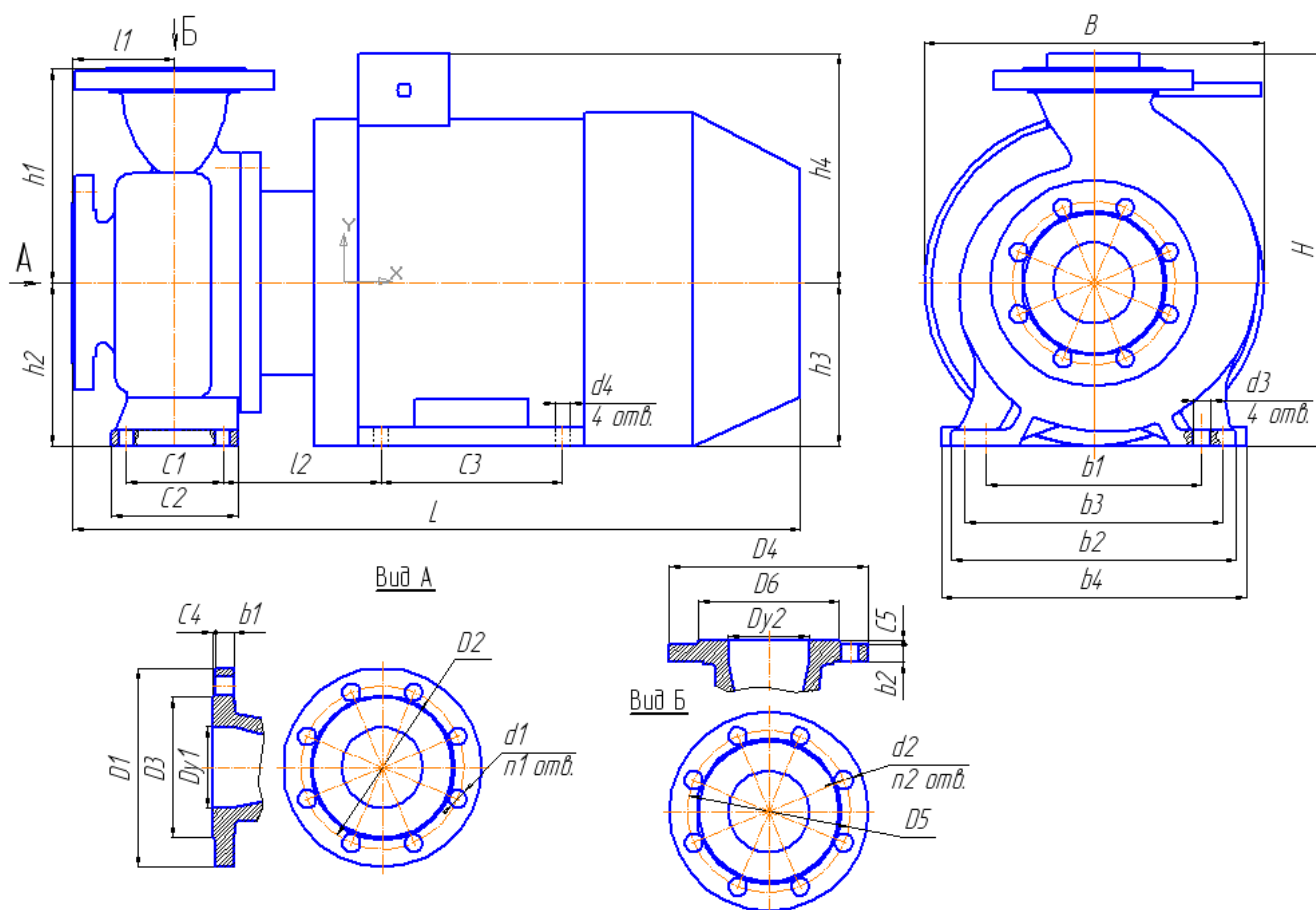
Рис. 5. Габаритные и присоединительные размеры Электронасоса Иртыш – ЦМК _____.
